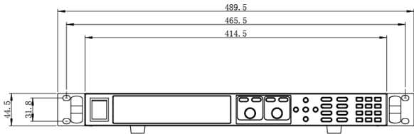
详细尺寸图
